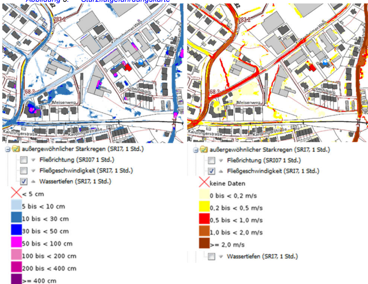
Abbildung 5: Sturzflutgefährdungskarte
