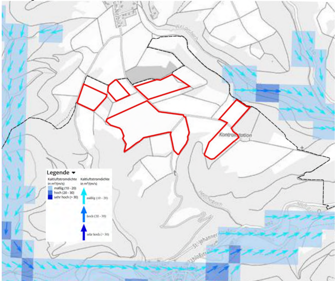
Abbildung 8: Kaltluftabfluss
