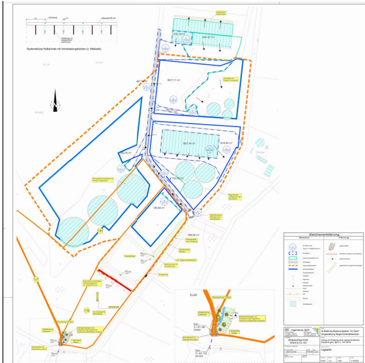
Abb.: Lageplan mit Darstellung des Entwässerungskonzeptes, Quelle Ingenieurbüro Brück und Saxler, Polcher Straße 4, 56727 Mayen
