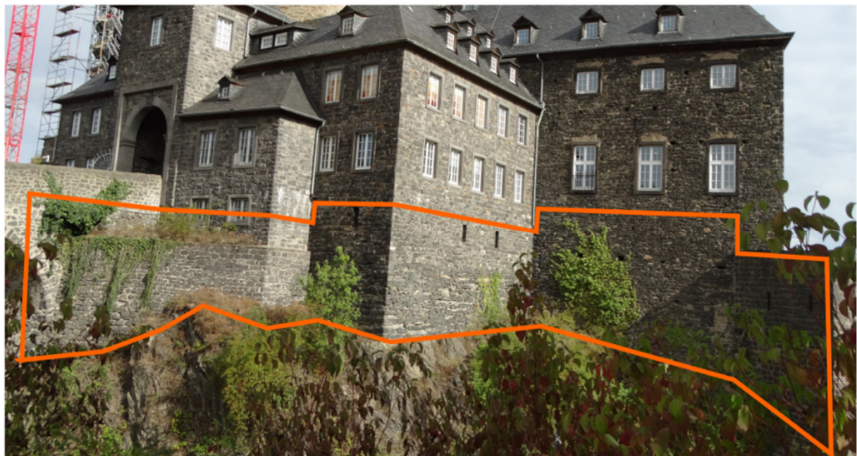
Ansicht Abschnitt 2
