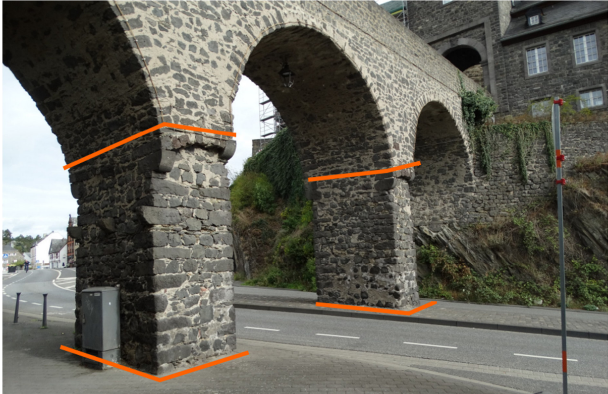
Ansicht Abschnitt 4. Die Pfeiler müssen umlaufend bearbeitet werden.
