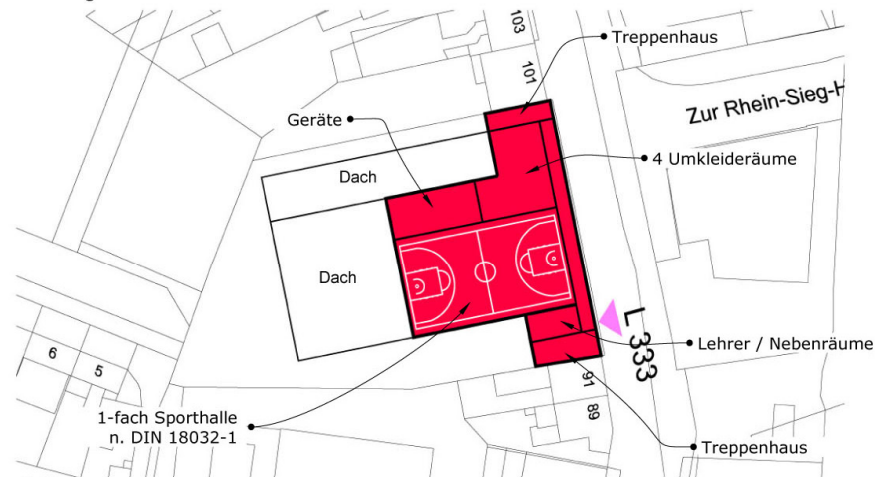
3.Obergeschoss
