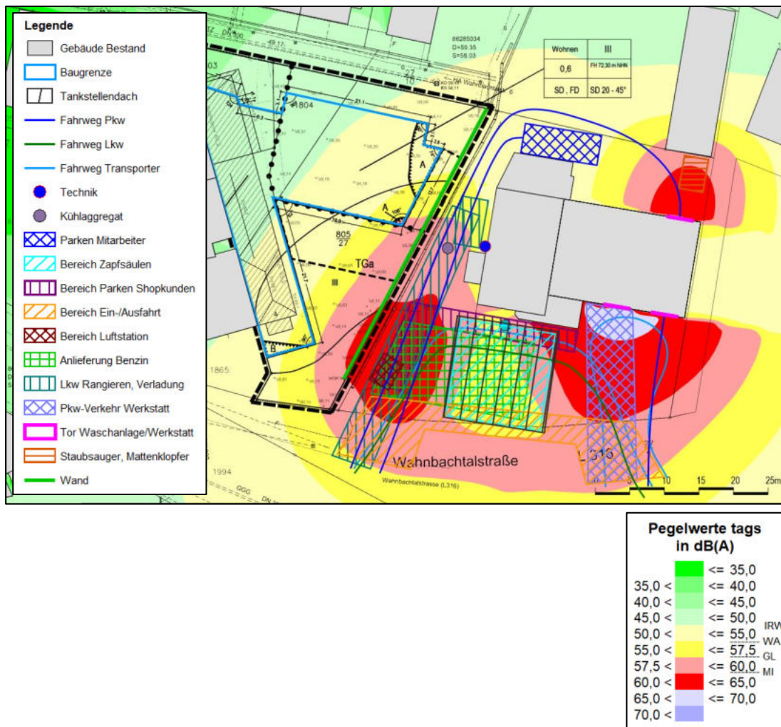
Abbildung 10 – Pegelverteilung Tankstelle tags
