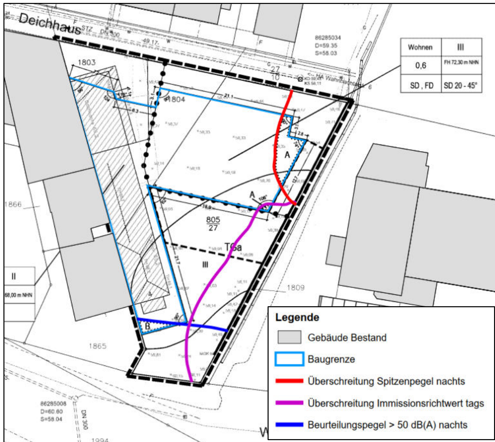
Abbildung 13 – Kennzeichnung der Bereiche für erforderliche Schallschutzmaßnahmen
