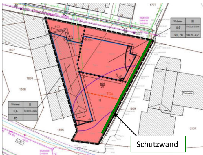
Abbildung 3 – Plangebiet und geplante Wand
