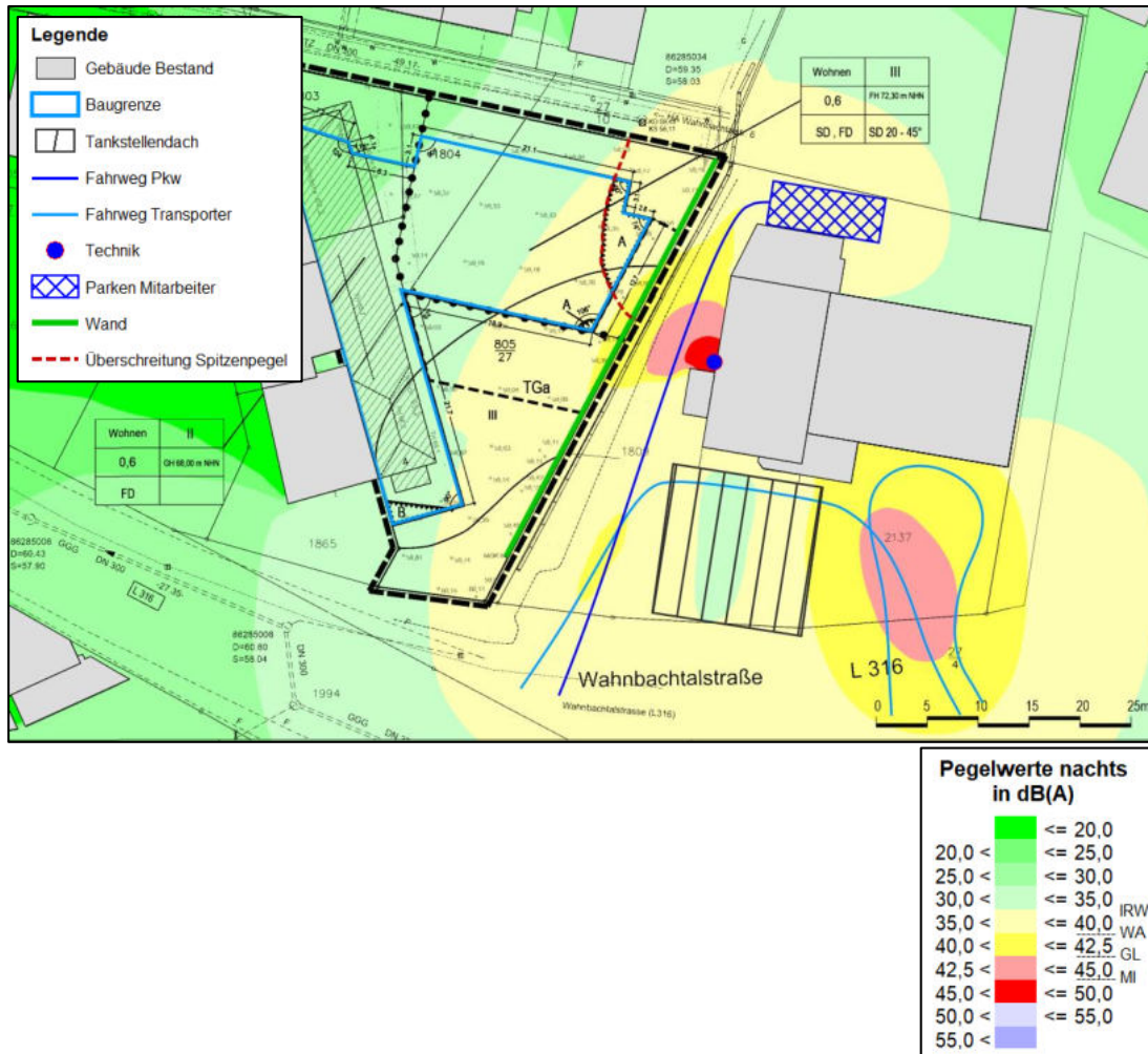
Abbildung 11 – Pegelverteilung Tankstelle nachts
