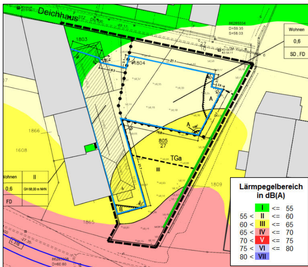
Abbildung 12 – Lärmpegelbereiche
