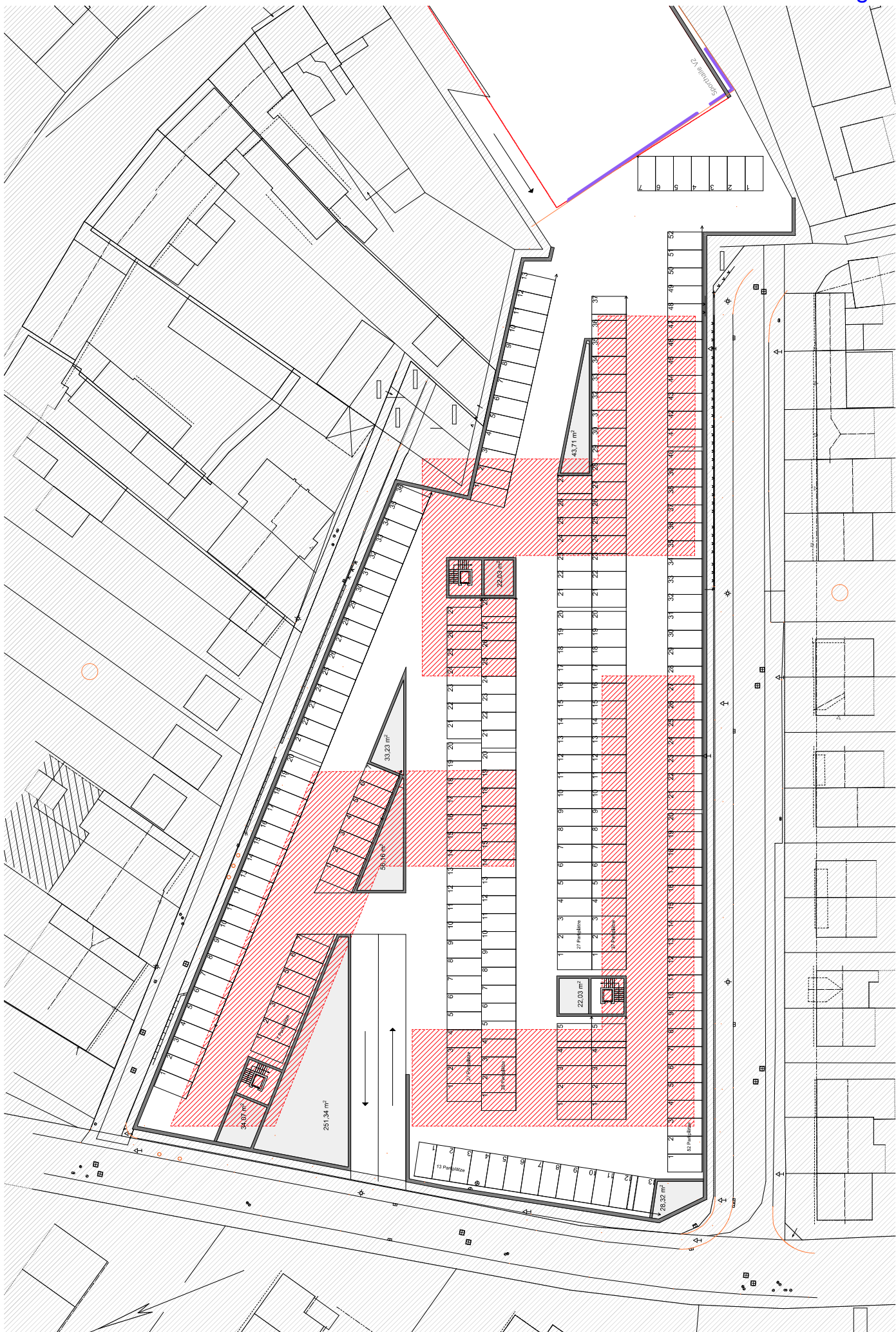
Tiefgarage 1:500
