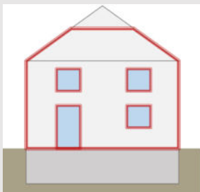
Darstellung der thermischen Gebäudehülle [eigene Darstellung]
