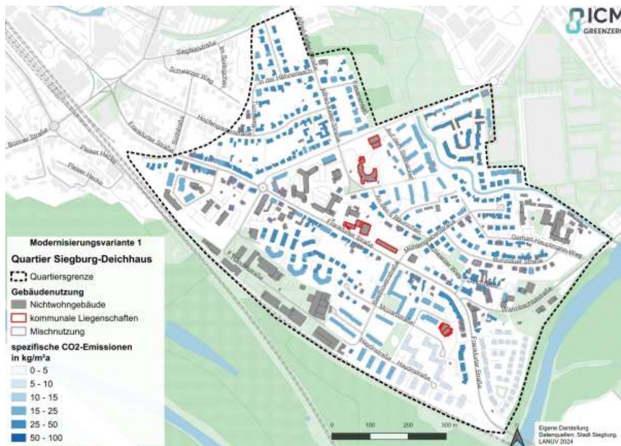
Abbildung 56: Spezifische CO 2 -Emissionen nach Umsetzung von Modernisierungsvariante 1
