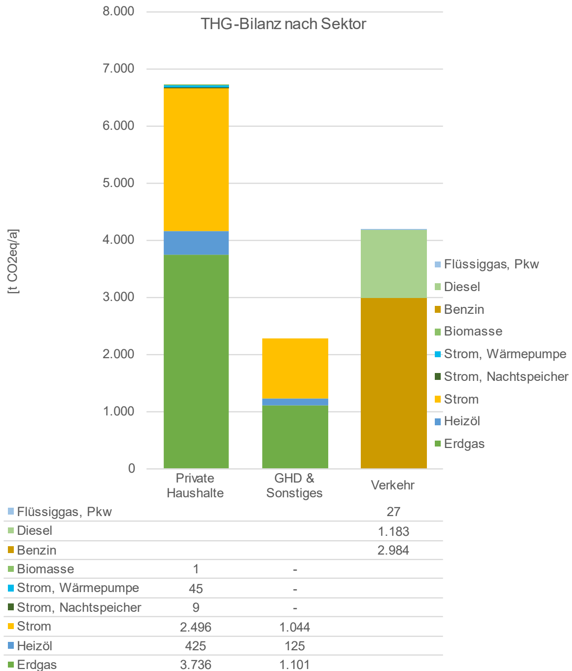
Abbildung 53: THG-Bilanz für das soziale Klimaquartier „Siegburg-Deichhaus“ Bilanzjahr 2022 (Die THG-Emissionen für Strom für Elektro-Pkw von 44 t CO 2 eq/a sind nicht im Diagramm berücksichtigt, da Anteile der Emissionen bereits in den bilanzierten Emissionen für Haushalte, GHD und Sonstiges enthalten sind)
