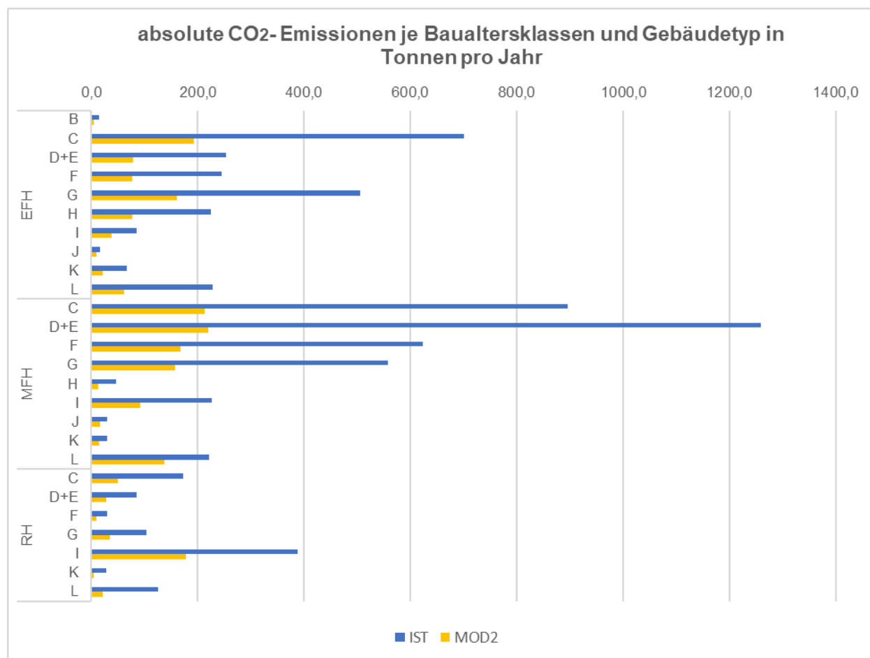
Abbildung 63: Gegenüberstellung der CO 2 -Emissionen von IST-Zustand und Modernisierungsvariante 2
