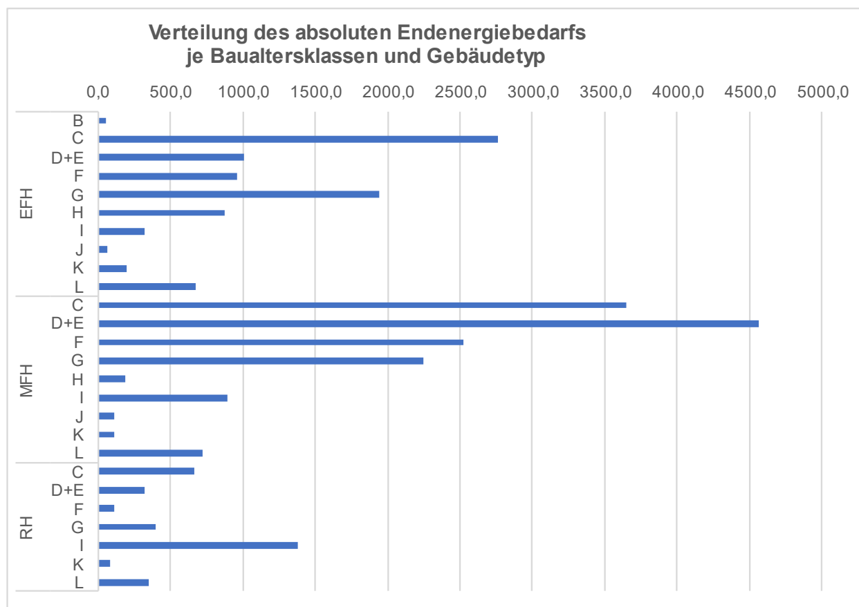
Abbildung 23: Verteilung des Endenergiebedarfs der Gebäudetypen pro Baualtersklasse in MWh/a
