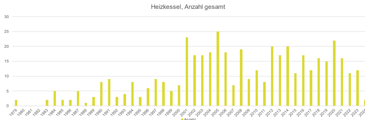
Abbildung 38: Heizkessel, Anzahl nach Baujahr
