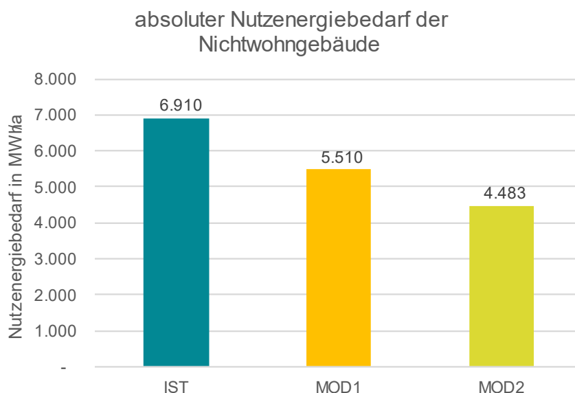
Abbildung 68: Nutzenergiebedarf des NWG-Bestands (Raumwärme, Trinkwarmwasser, Prozesswärme; eigene Berechnung nach LANUV 26 Daten KWP)
