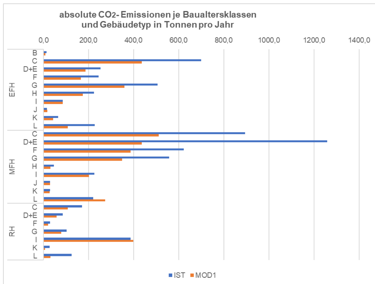
Abbildung 58: Gegenüberstellung der CO 2 -Emissionen von IST-Zustand und Modernisierungsvariante 1
