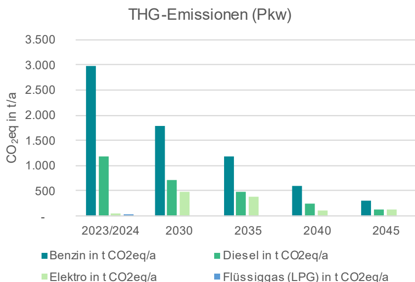
Abbildung 91: THG-Emissionen für Pkw nach Kraftstoffart / Energieträger bis 2045 50
