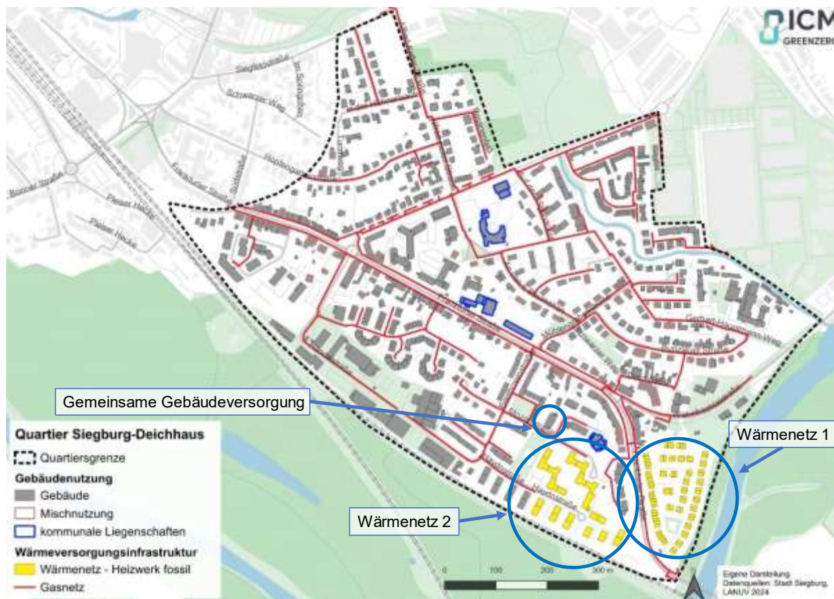
Abbildung 34: Darstellung der Wärmeversorgungsinfrastruktur
