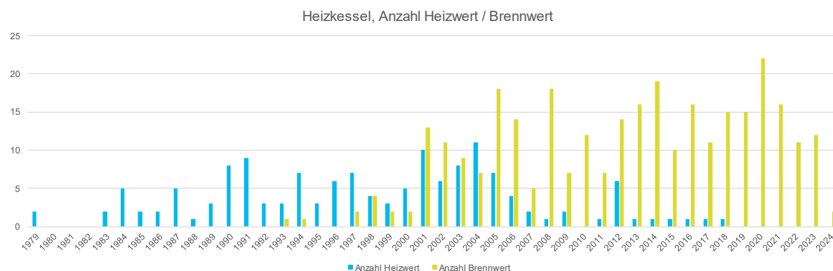
Abbildung 40: Heizkessel, Anzahl Heizwert / Brennwert je Baujahr
