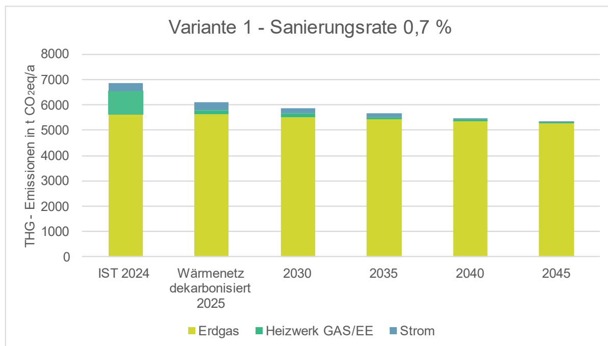
Abbildung 84: THG-Emissionen bei einer Annahme der Sanierungsrate im Wohngebäudebereich von 0,7 % und Modernisierungsvariante MOD2, THG-Faktoren nach KEA-WP Technikkatalog Kommunale Wärmeplanung. Grün-schraffiert = THG-Emissionen der fossilen Wärmenetzversorgung (Heizwerk Gas)
