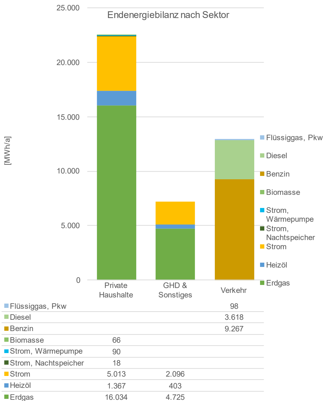
Abbildung 51: Endenergiebilanz für das soziale Klimaquartier „Siegburg-Deichhaus“ Bilanzjahr 2022 (Der Stromverbrauch an Endenergie für Elektro-Pkw von 100 MWh/a ist nicht im Diagramm berücksichtigt, da Anteile des Stromverbrauchs bereits im bilanzierten Stromverbrauch für Haushalte, GHD und Sonstiges enthalten sind)
