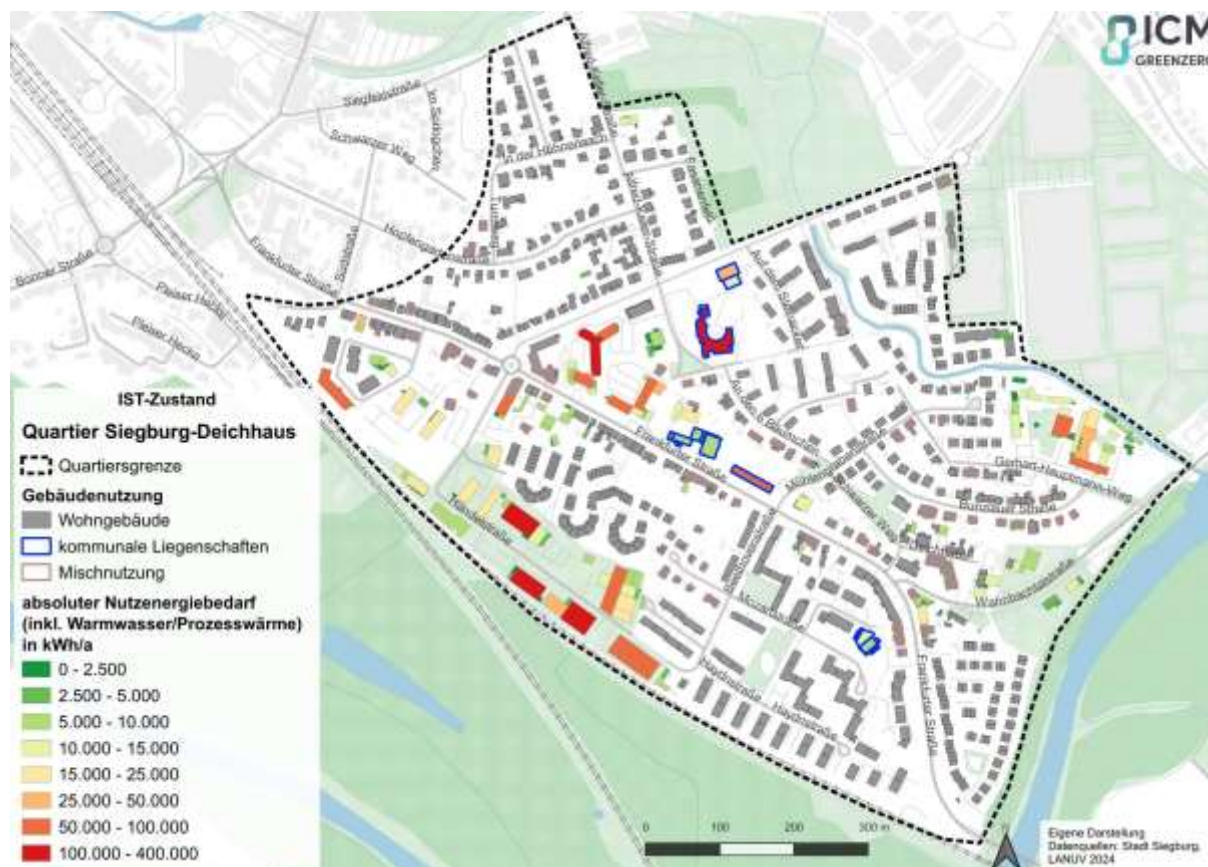
Abbildung 28: Darstellung des absoluten Nutzenergiebedarfs des NWG-Bestandes
