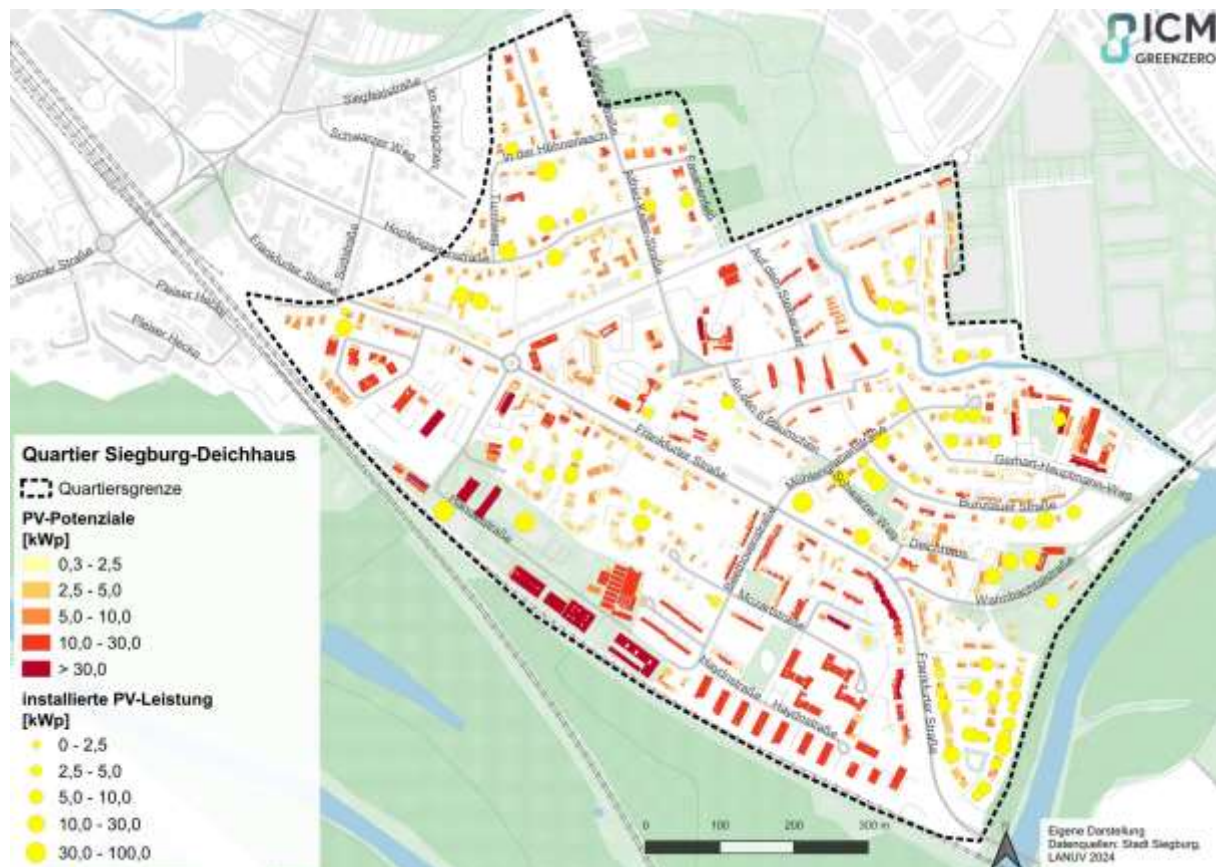
Abbildung 75: Darstellung der räumlichen Verteilung des theoretischen PV-Aufdach-Potenzials mit den aktuell installierten PV-Anlagen
