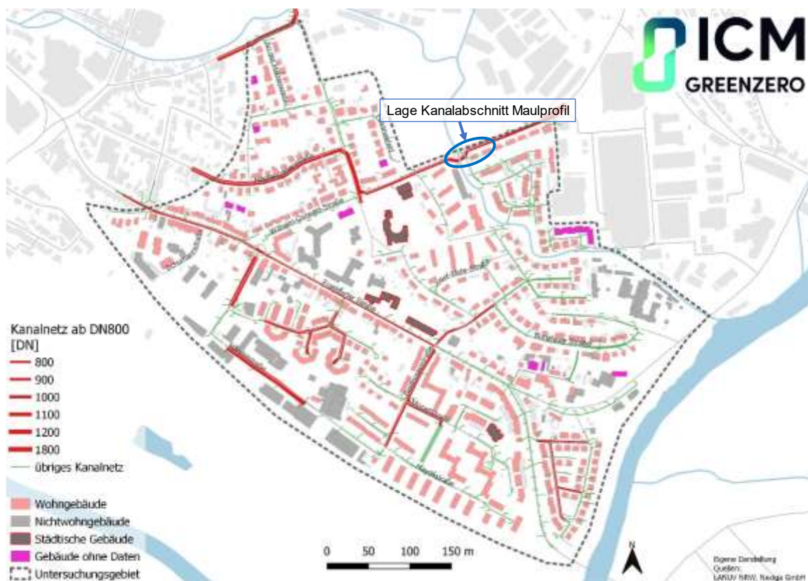
Abbildung 81: Kanalnetz im Quartier Deichhaus, rot hervorgehoben, Kanalquerschnitte > DN800. (Quelle: Eigene Darstellung)
