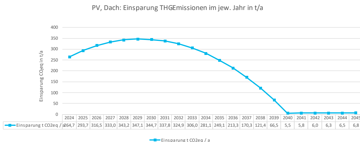
Abbildung 89: Einsparung THG-Emissionen durch Aufdach-Photovoltaik für die jeweiligen Jahre bis 2045
