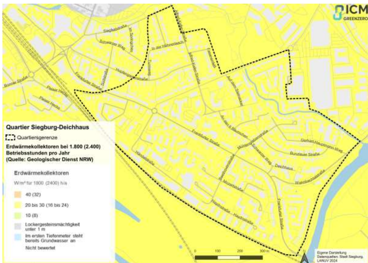
Abbildung 76: Darstellung der Entzugsleistung von Erdwärmekollektoren in W/m 2
