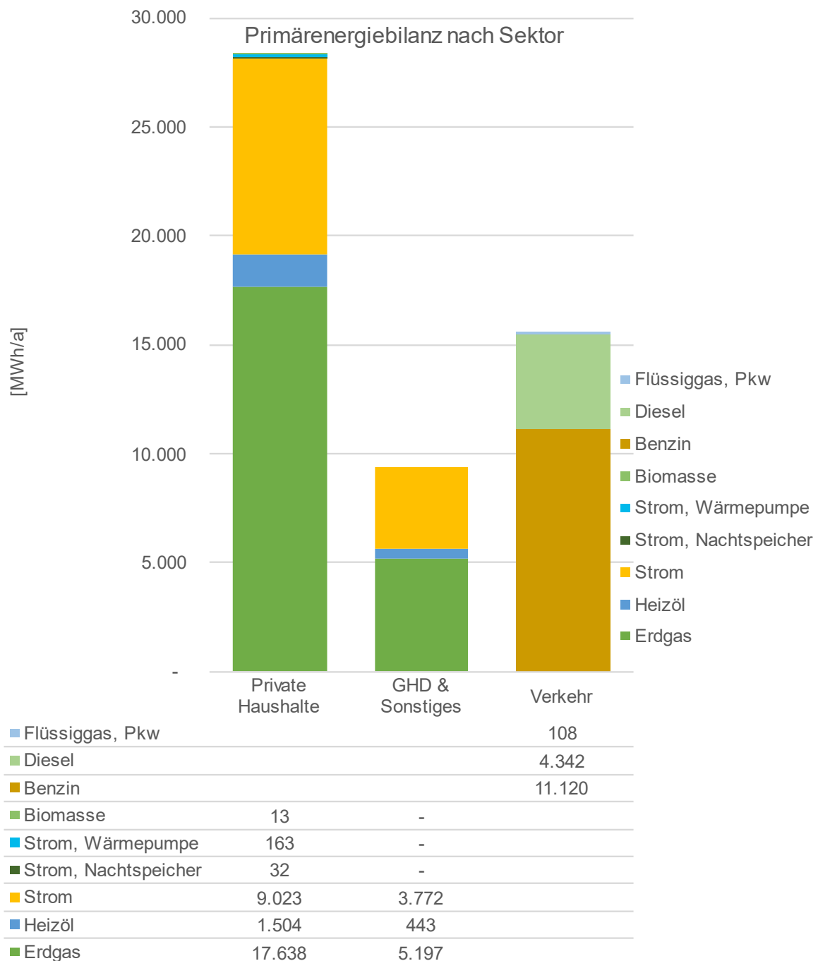
Abbildung 52: Primärenergiebilanz für das soziale Klimaquartier „Siegburg-Deichhaus“ Bilanzjahr 2022 (Der Stromverbrauch an Primärenergie für Elektro-Pkw von 180 MWh/a ist nicht im Diagramm berücksichtigt, da Anteile des Stromverbrauchs bereits im bilanzierten Stromverbrauch für Haushalte, GHD und Sonstiges enthalten sind)
