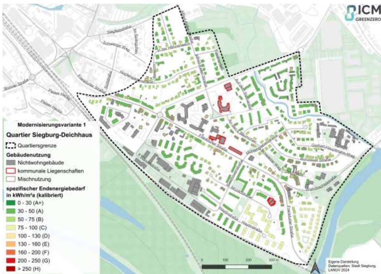
Abbildung 54: Darstellung des spezifischen auf typische Verbrauchswerte kalibrierten Endenergiebedarfs des Wohngebäudebestands nach Umsetzung der Modernisierungsvariante 1
