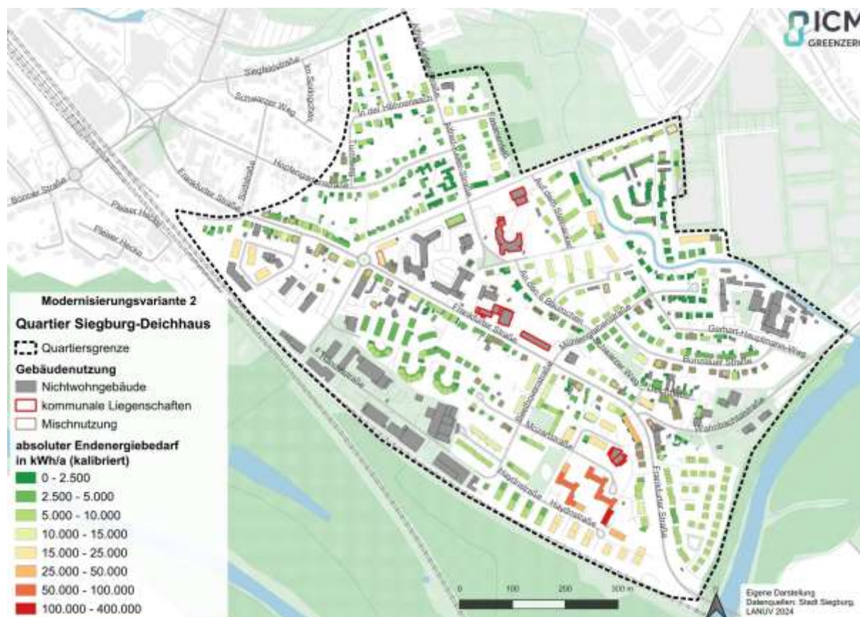
Abbildung 60: Darstellung des absoluten auf typische Verbrauchswerte kalibrierten Endenergiebedarfs des Wohngebäudebestands nach Umsetzung der Modernisierungsvariante 2
