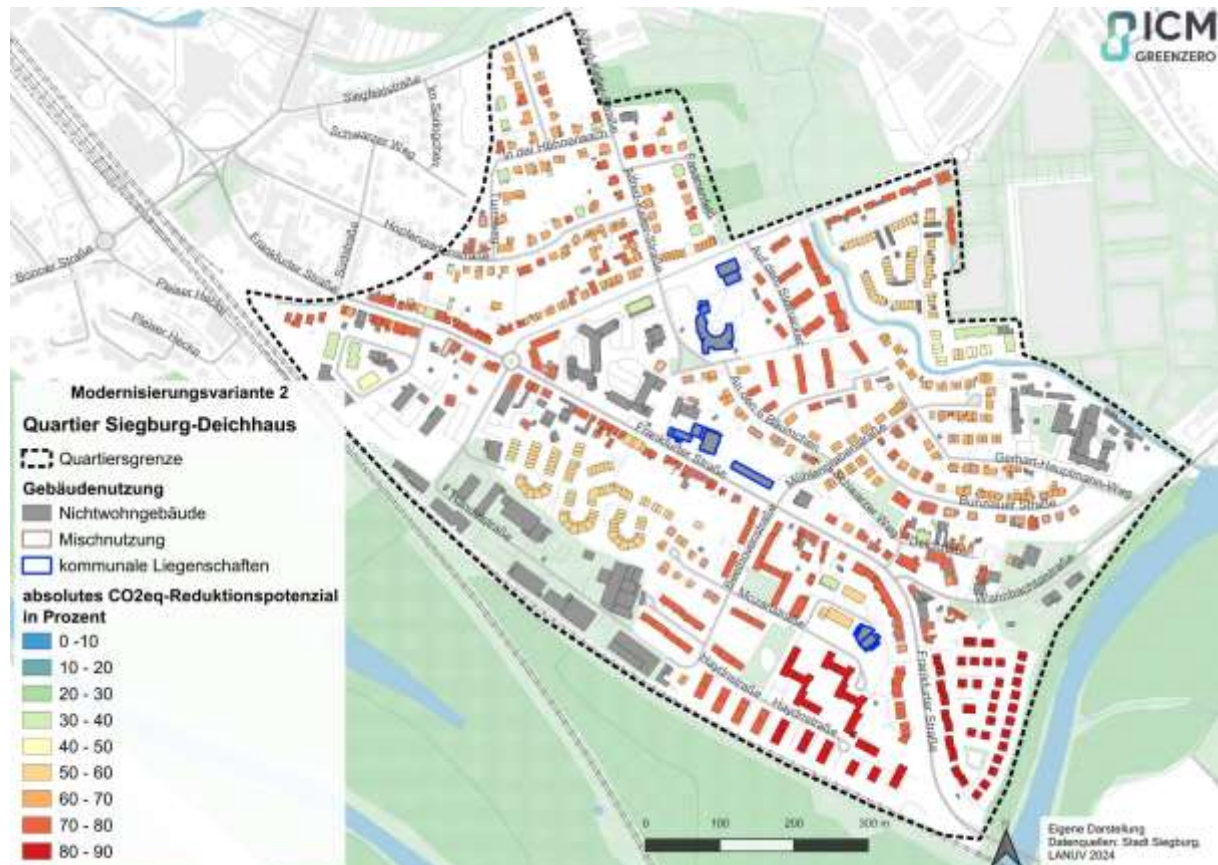
Abbildung 62: Darstellung des prozentualen CO 2 -Reduktionspotenzials nach Umsetzung von Modernisierungsvariante 2
