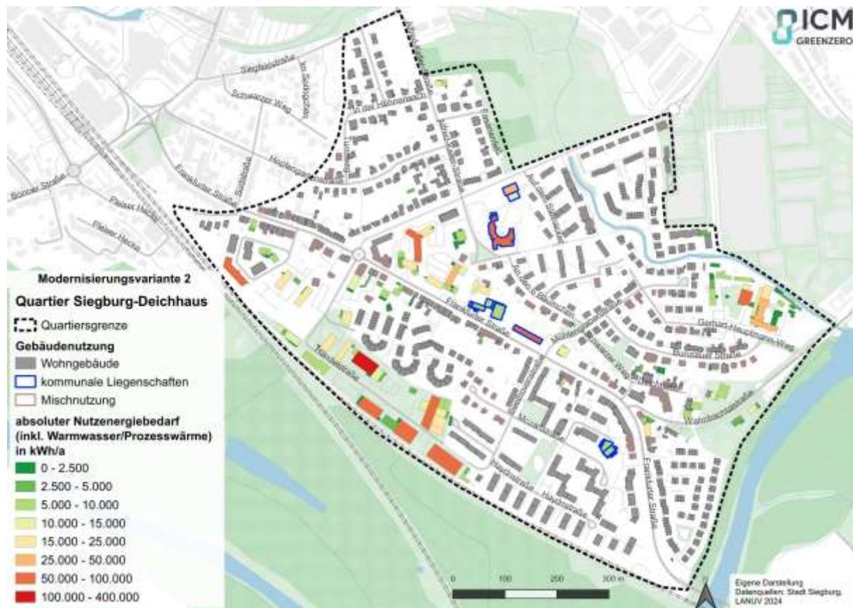
Abbildung 67: Darstellung des absoluten Nutzenergiebedarfs des NWG-Bestands nach Modernisierungsvariante 2
