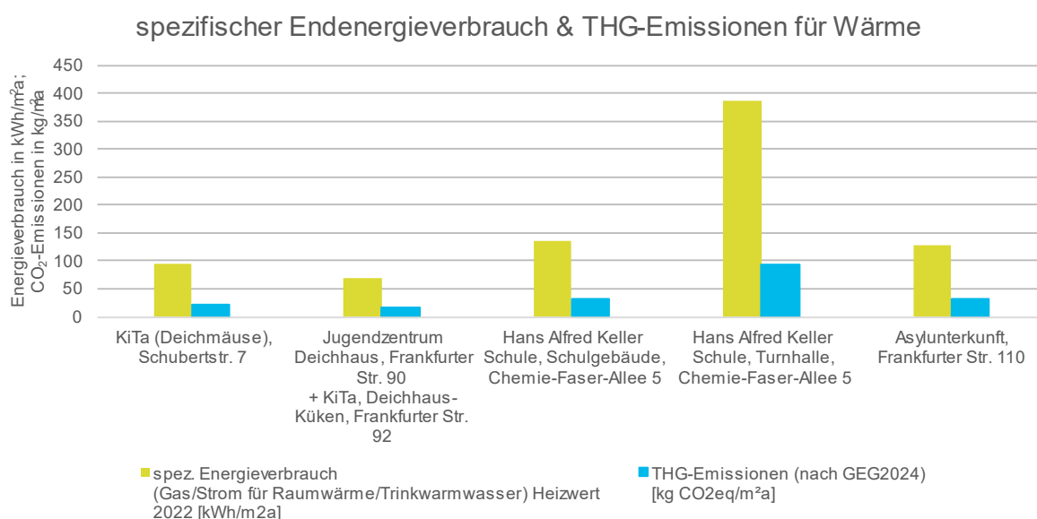
Abbildung 29: Auswertung der Energieverbräuche der kommunalen Nichtwohngebäude im Quartier für das 2022
