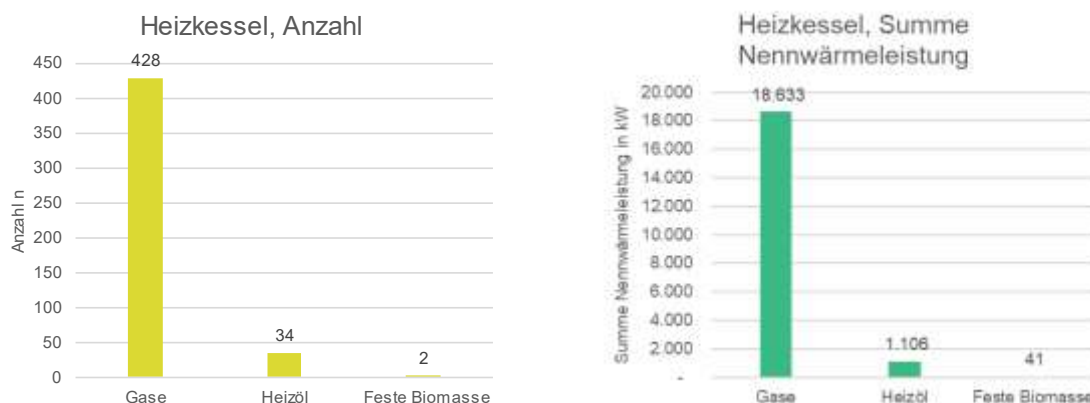
Abbildung 37: Heizkessel, Anzahl und Summe der Nennwärmeleistung nach Energieträger
