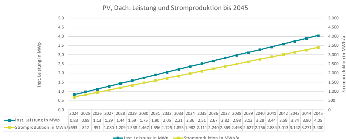
Abbildung 88: Installierte PV-Leistung (Aufdach) und Stromproduktion für die Jahre bis 2045
