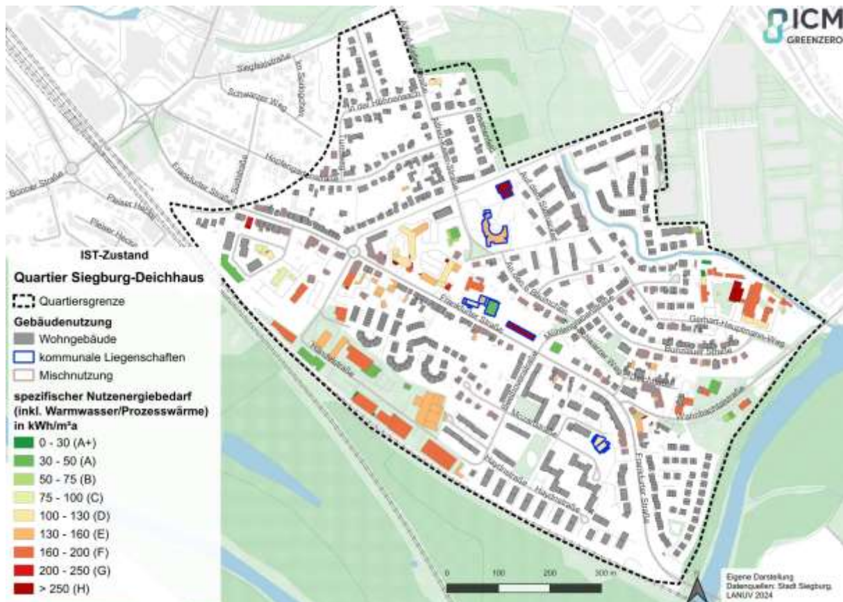
Abbildung 27: Darstellung des spezifischen Nutzenergiebedarfs des NWG-Bestandes
