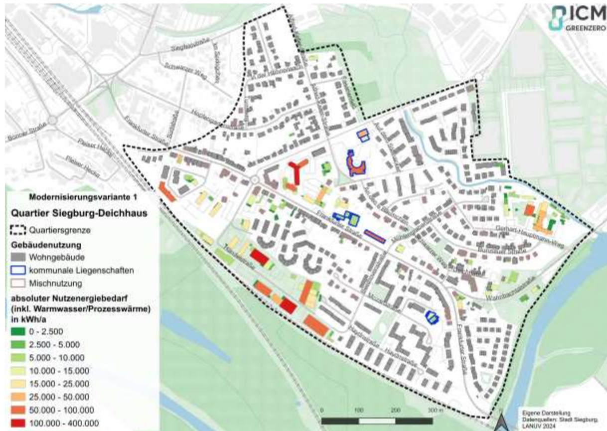
Abbildung 65: Darstellung des absoluten Nutzenergiebedarfs des NWG-Bestands nach Modernisierungsvariante 1
