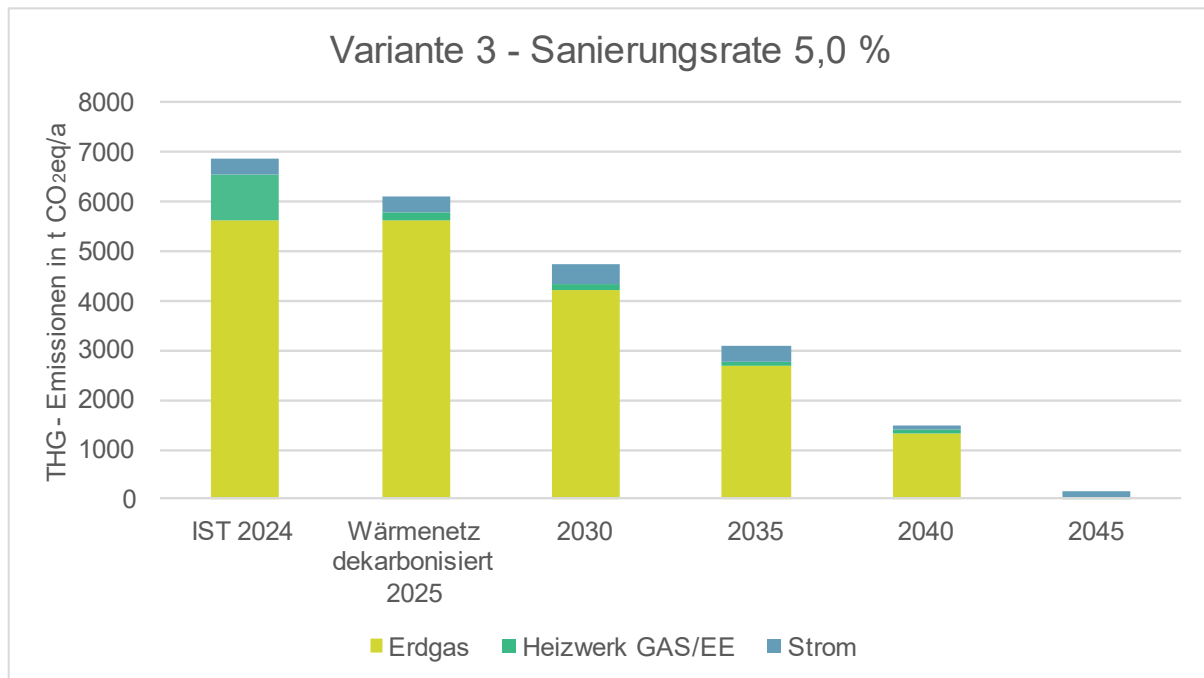
Abbildung 86: THG-Emissionen bei einer Annahme der Sanierungsrate im Wohngebäudebereich von 5 % und Modernisierungsvariante MOD2, THG-Faktoren nach KEA-WP Technikkatalog Kommunale Wärmeplanung. Grün-schraffiert = THG-Emissionen der fossilen Wärmenetzversorgung (Heizwerk Gas)
