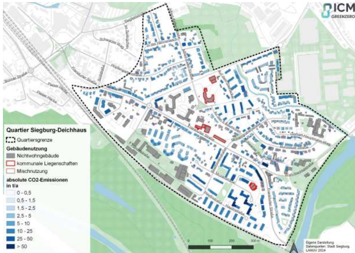
Abbildung 25: Absolute CO 2 -Emissionen des Wohngebäudebestandes (CO 2 -Faktoren nach GEG 2024)
