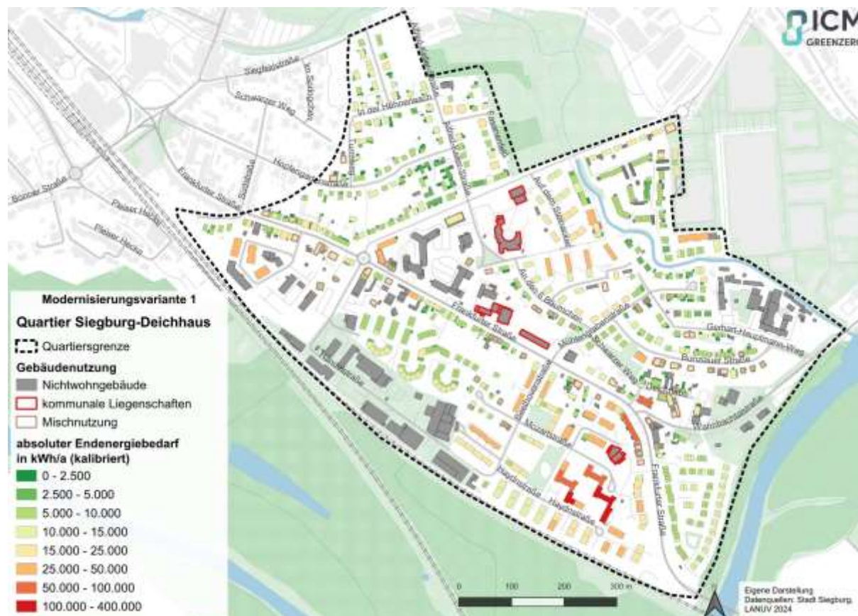
Abbildung 55: Darstellung des absoluten auf typische Verbrauchswerte kalibrierten Endenergiebedarfs des Wohngebäudebestands nach Umsetzung der Modernisierungsvariante 1
