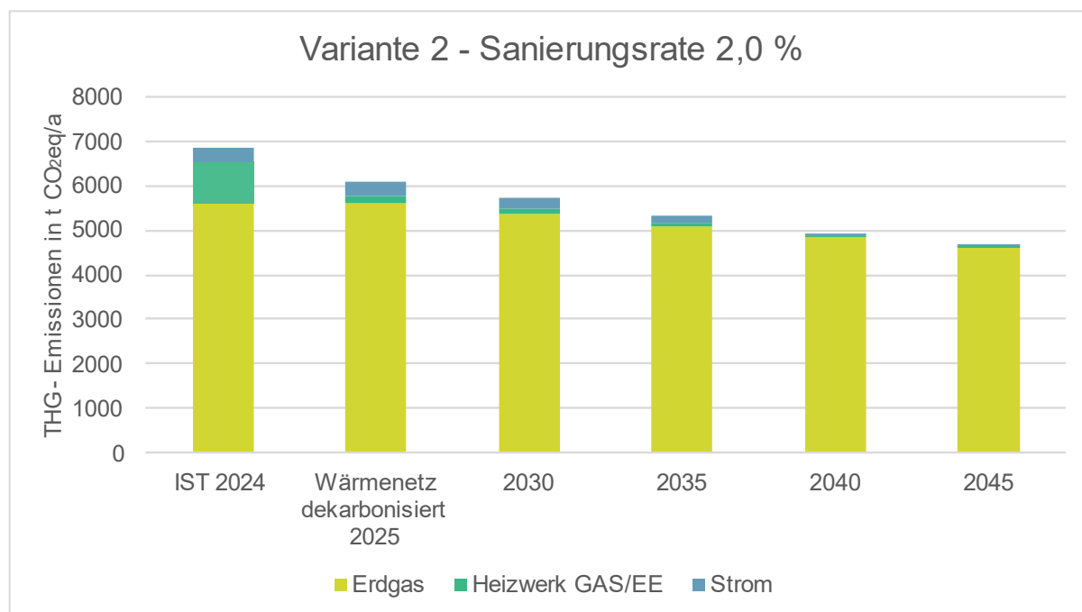
Abbildung 85: THG-Emissionen bei einer Annahme der Sanierungsrate im Wohngebäudebereich von 2 % und Modernisierungsvariante MOD2, THG-Faktoren nach KEA-WP Technikkatalog Kommunale Wärmeplanung. Grün-schraffiert = THG-Emissionen der fossilen Wärmenetzversorgung (Heizwerk Gas)
