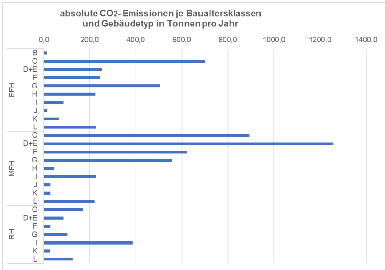
Abbildung 26: Absolute CO 2 -Emissionen der Gebäudetypen pro Baualtersklasse
