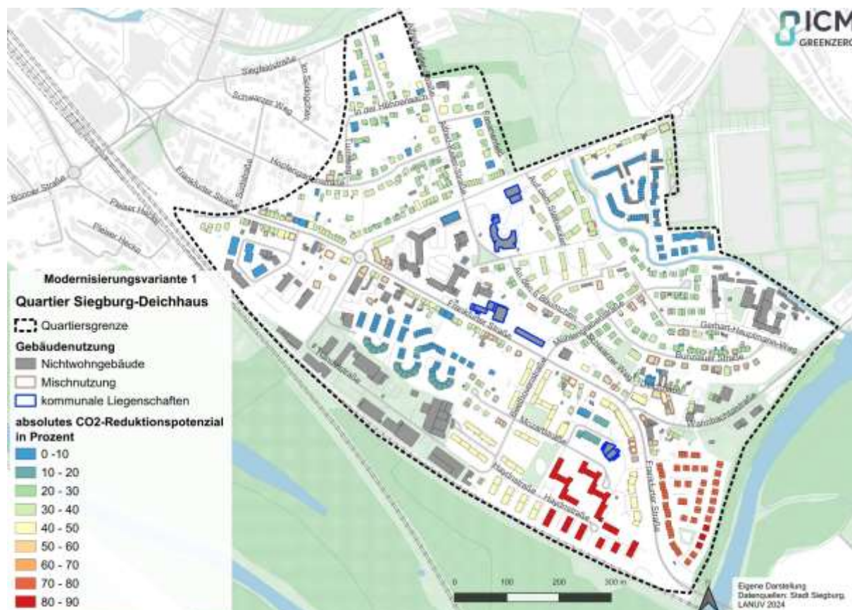
Abbildung 57: Darstellung des prozentualen CO 2 -Reduktionspotenzials nach Umsetzung von Modernisierungsvariante 1
