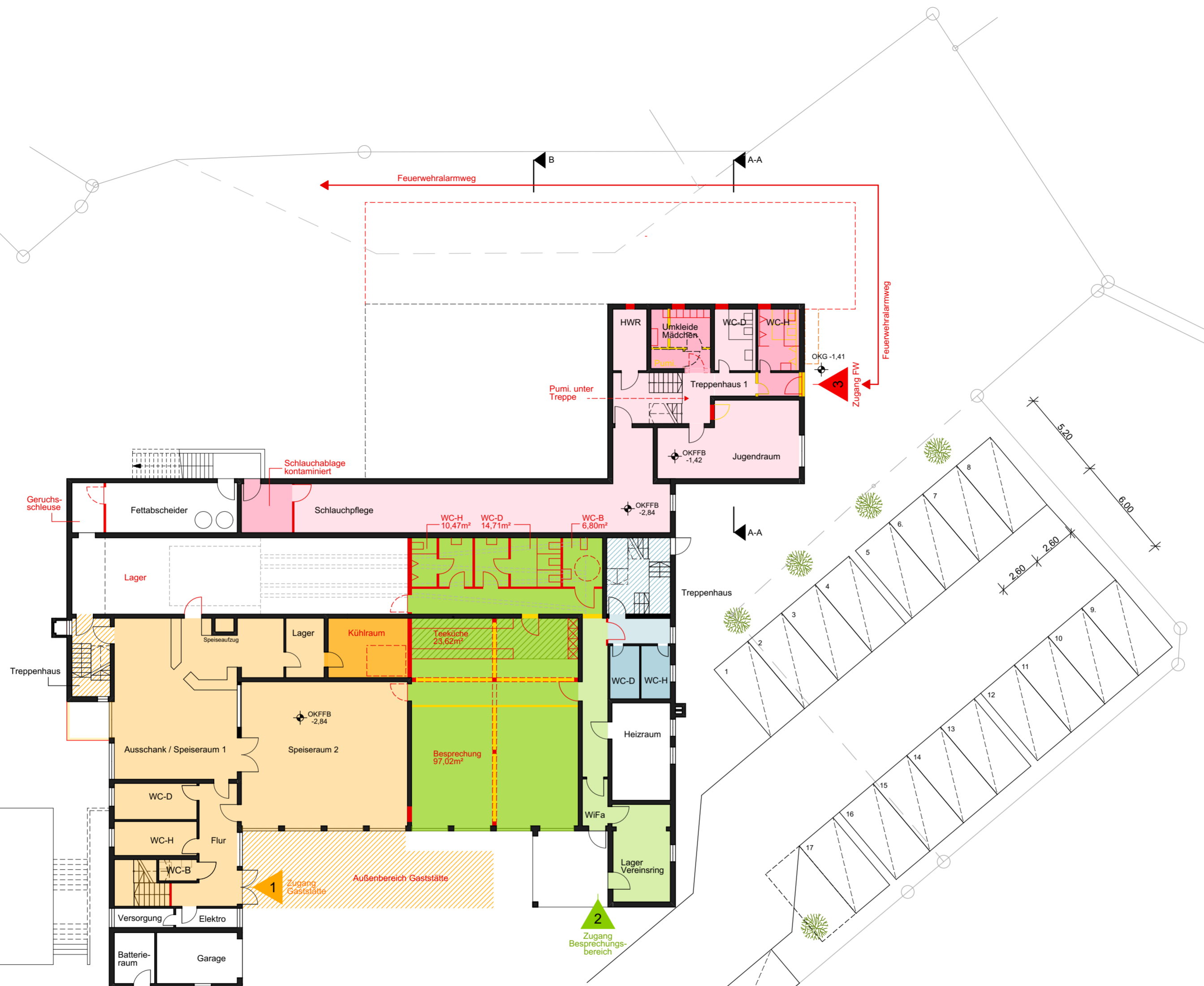
Grundriss Ebene UG
