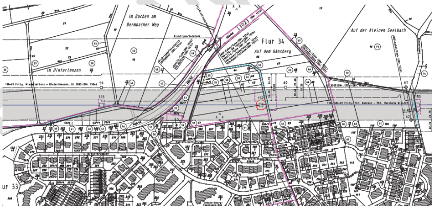
Abbildung 4: Ausschnitt aus dem Lageplan Register 6.1.31, Bl. 39
