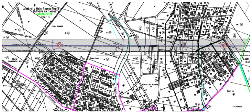
Abbildung 8: Ausschnitt aus dem Lageplan Register 6.1.38.
