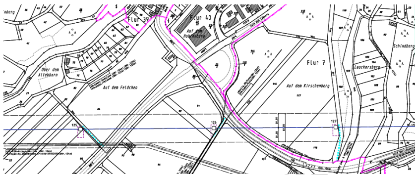
Abbildung 1: Ausschnitt aus dem Lageplan Register 6.1.27 – Blatt 33.1
